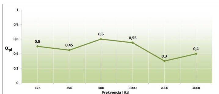
Priebeh činiteľa zvukovej pohltivosti pre OBIFON Acutone
