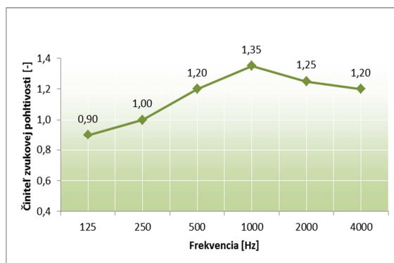
Priebeh činiteľa zvukovej pohltivosti pre OBIFON Diffсорber
